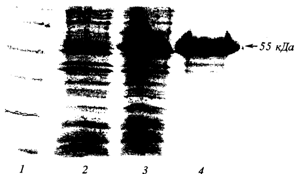
Рис. 3. Бактериальная экспрессия рекомбинантного белка DDBA3: 1 — маркер молекулярной массы LMW («Amersham Pharmacia Biotech.»); 2 — суммарные бактериальные белки до индукции; 3 — суммарные бактериальные белки после индукции; 4 — очищенные белковые тельца включения
