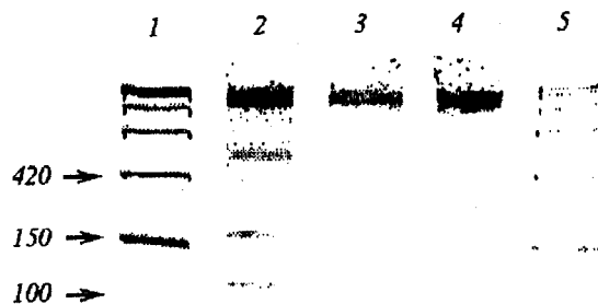
Рис. 5. Детекция мутаций в dbl области bcr/abl гена методом химического расщепления ДНК-ДНК гетеродуплексов: 1, 5 — маркер молекулярной массы PCR marker («Promega», США); 2 — химическое расщепление гетеродуплексов А. + К. с образованием продуктов размером 420, 250 и 100 п. н.; 3, 4 — нерасщепленные гетеродуплексы А. + Ф. и А. + K562 соответственно
