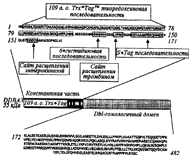
Рис. 6. Схема рекомбинантного белка DDBA3
